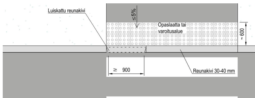
Reumatuen asennus suojatien kohdalla. (Lähde: SuRaKu ohjekortti 1/7.)
