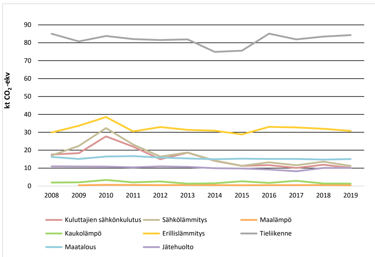
Kuva 16. Sektorikohtaisten päästöjen kehitys Vihdissä vuosina 2008–2019. Vuoden 2019 tiedot perustuvat osittain ennakkotietoihin.
