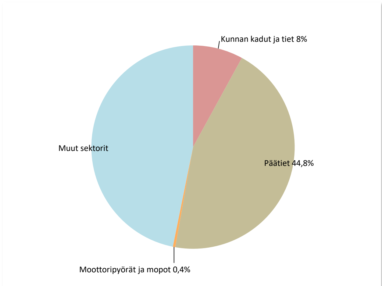
Kuva 7. Tieliikenteen päästöjen osuus kokonaispäästöistä (ilman teollisuutta) Vihdissä vuonna 2020 ja sektorin jakautuminen eri päästölähteisiin.
