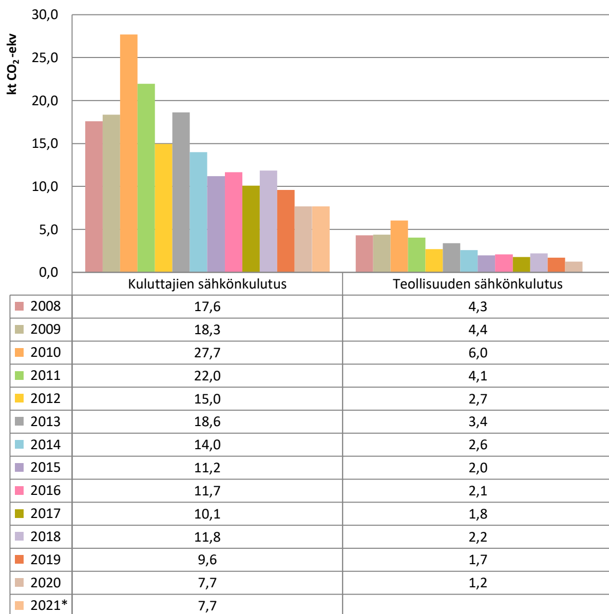
Kuva 3. Kuluttajien ja teollisuuden sähkönkulutuksen päästöjen kehitys Vihdissä vuosina 2008–2021. Vuoden 2021 tieto on ennakkotieto. Sitä ei ole esitetty teollisuuden sähkönkulutukselle.
