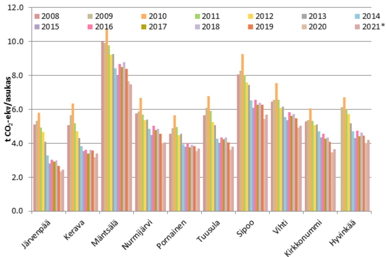
Kuva 21. KUUMA-kuntien asukaskohtaisten päästöjen kehitys vuosina 2008–2021 ilman teollisuutta. Vuoden 2021 tieto on ennakkotieto.
