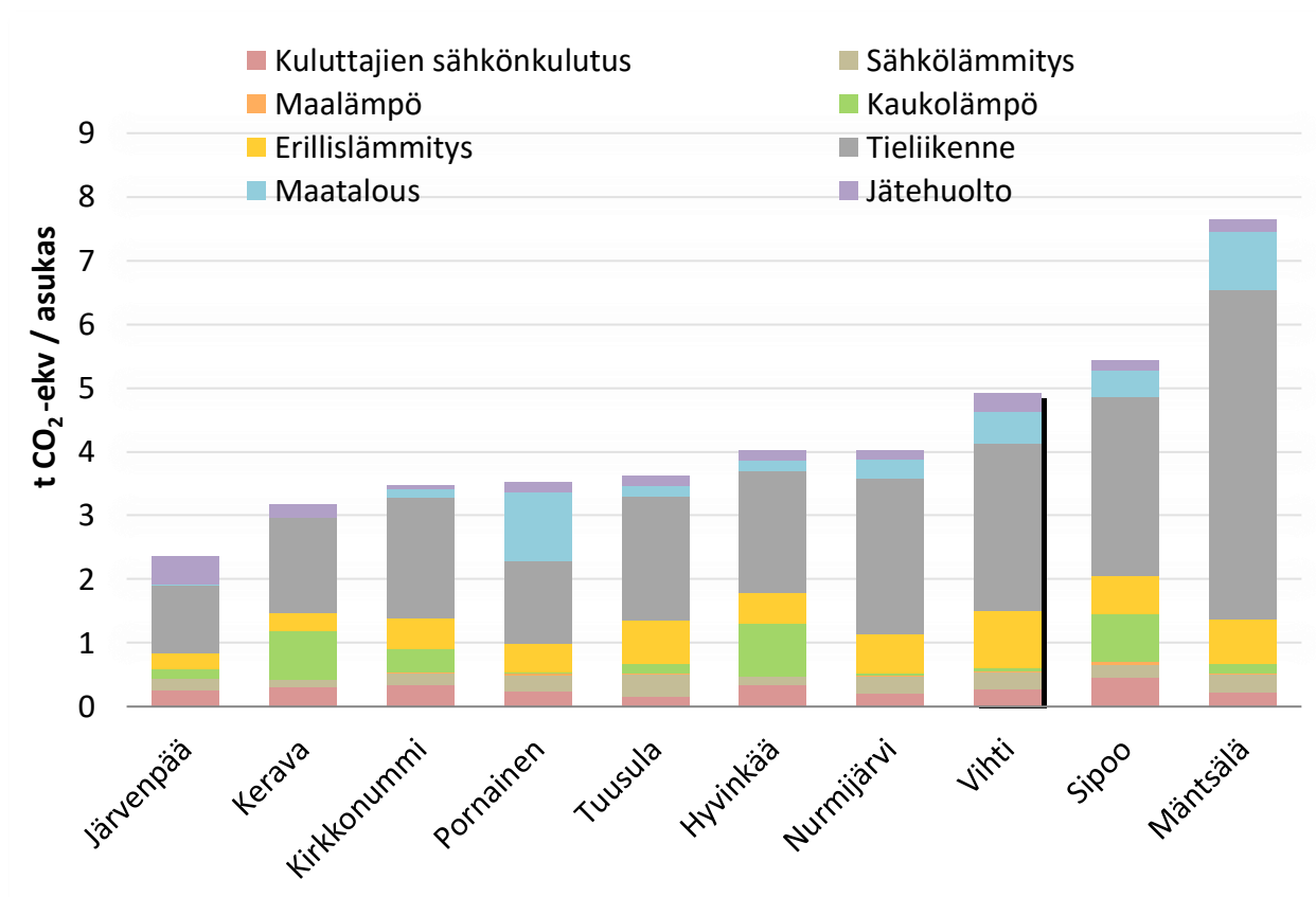
Kuva 22. KUUMA-kuntien asukaskohtaiset päästöt sektoreittain vuonna 2020.
