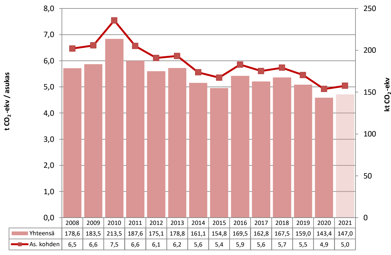
Kuva 16. Päästöt yhteensä ja asukasta kohden Vihdissä vuosina 2008–2021 ilman teollisuutta. Vuoden 2021 tieto on ennakkotieto.
