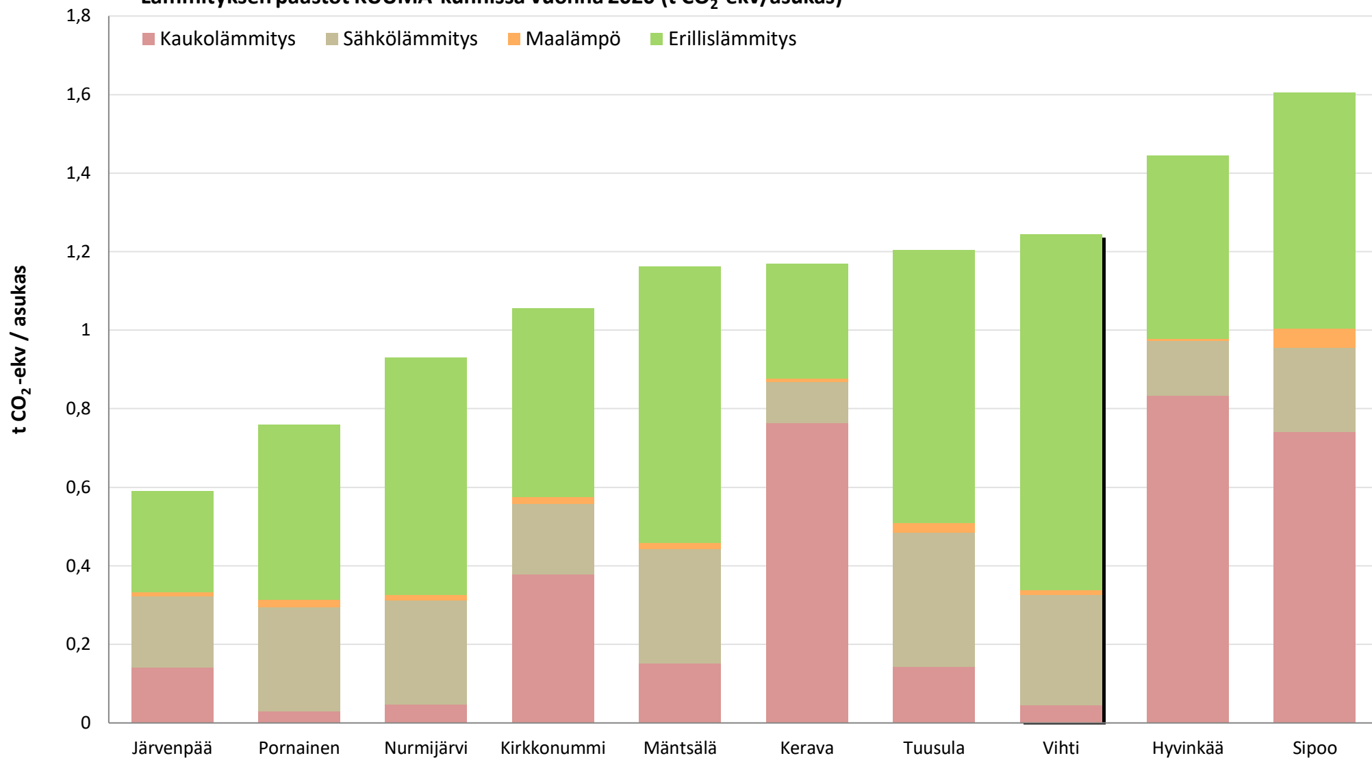
Lämmityksen päästöt KUUMA-kunnissa vuonna 2020 (t CO 2 -ekv/asukas)
