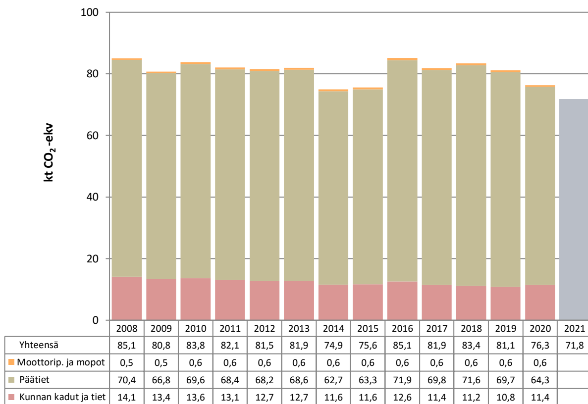
Kuva 8. Tieliikenteen päästöt Vihdissä vuosina 2008–2021. Vuoden 2021 tieto on ennakkotieto, joka perustuu liikennemäärien muutoksiin kunnan alueella.
