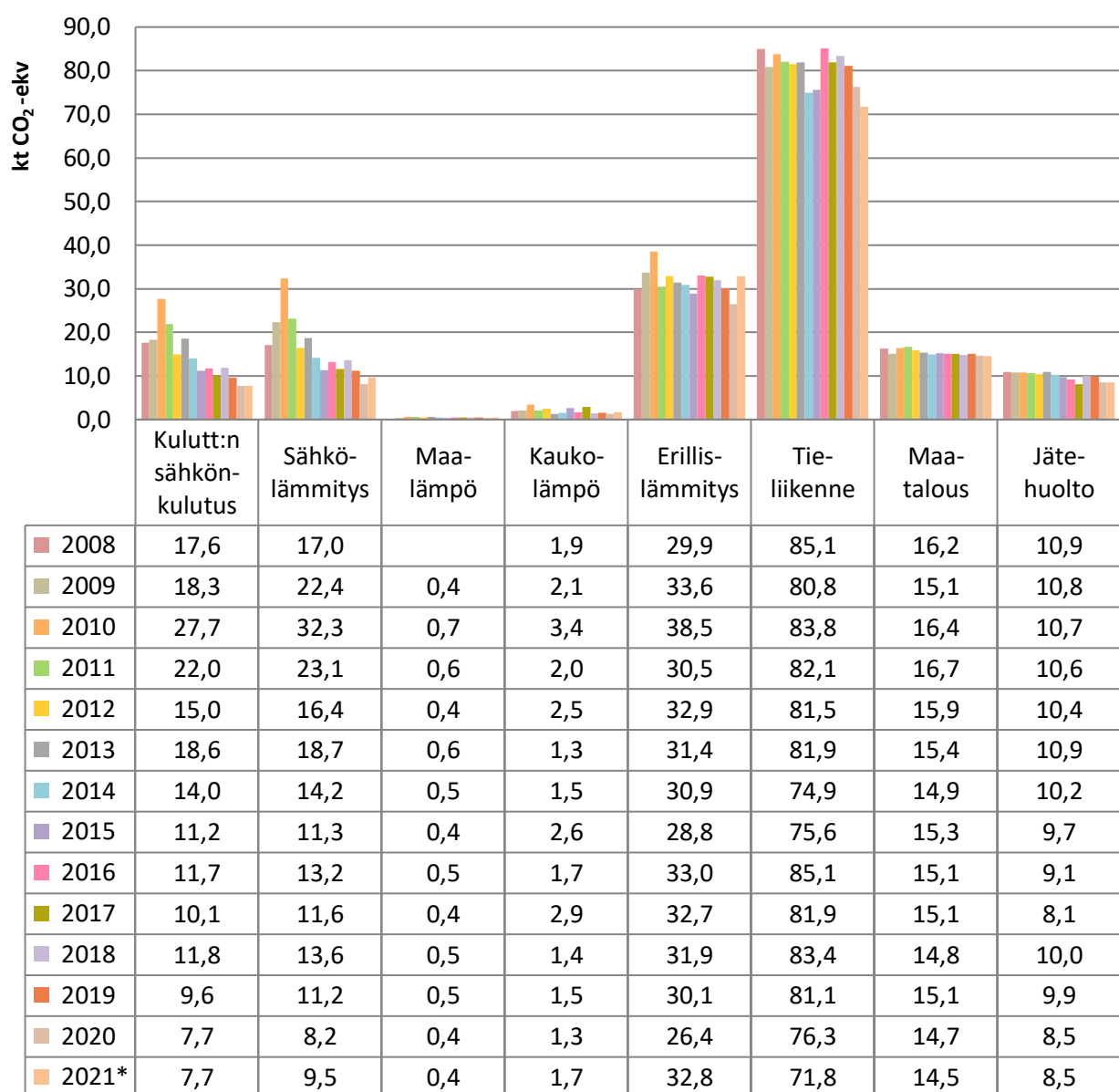
Kuva 14. Päästöt sektoreittain Vihdissä vuosina 2008–2021 ilman teollisuutta. Vuoden 2021 tieto on ennakkotieto.
