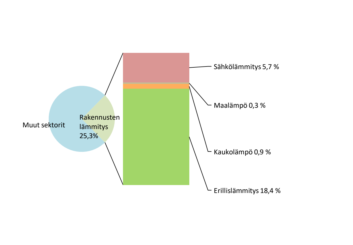
Kuva 5. Rakennusten lämmityksen päästöjen osuus kokonaispäästöistä (ilman teollisuutta) Vihdissä vuonna 2020 ja sektorin jakautuminen eri päästölähteisiin.
