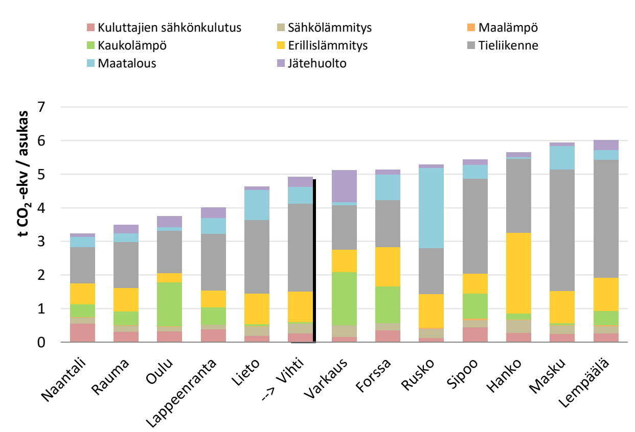
Kuva 20. Asukaskohtaisten päästöjen vertailu (ilman teollisuutta) vuonna 2020 sellaisissa CO2-raportin kunnissa, joissa on 50–100 asukasta maaneliökilometrillä.
