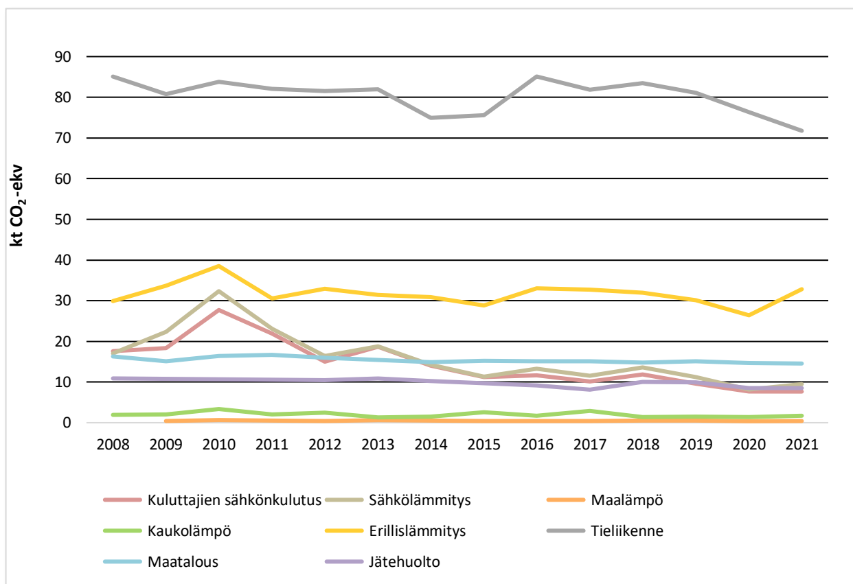
Kuva 15. Sektorikohtaisten päästöjen kehitys Vihdissä vuosina 2008–2021. Vuoden 2021 tiedot perustuvat osittain ennakkotietoihin.
