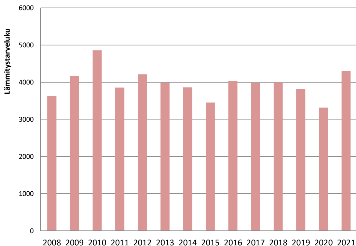
Kuva 4. Vihdin lämmitystarveluvut vuosina 2008–2021.
