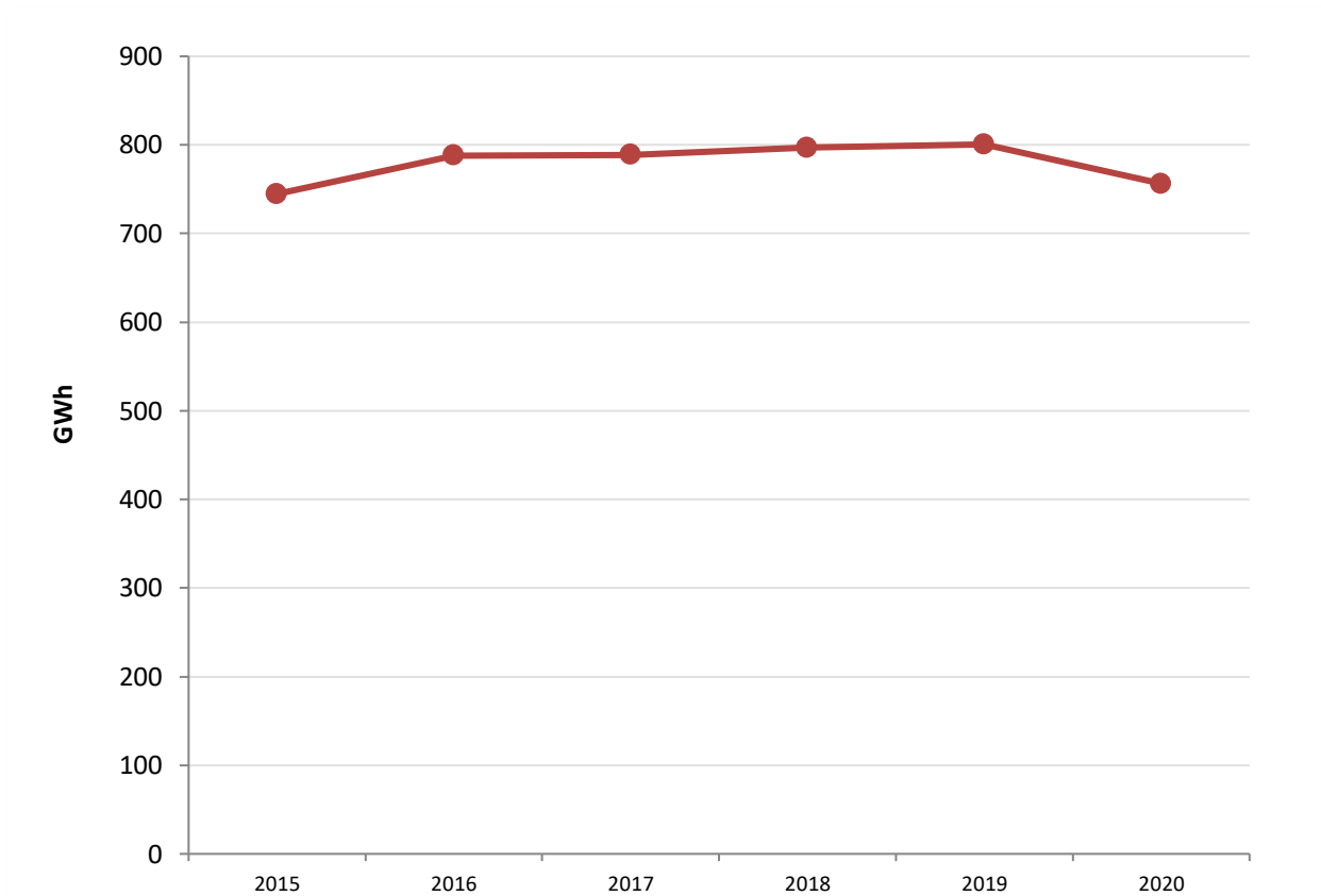
Kuva 24. Energian loppukulutuksen kehitys Vihdissä vuosina 2015–2020 ilman teollisuutta. Energian loppukulutus ei sisällä lämpöpumppujen tuottamaa uusiutuvaa energiaa, mutta sisältää niiden käyttämän sähkön.
