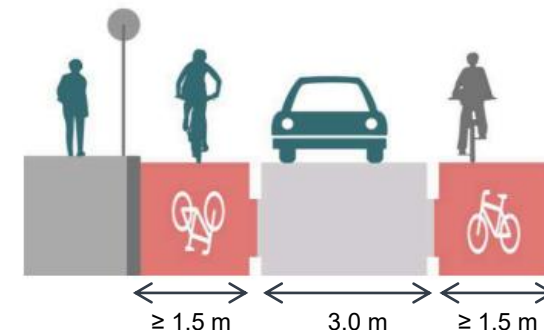
2-1 -tie pyöräkaistamerkinnällä (rakennetun ympäristön kylätieratkaisu)
