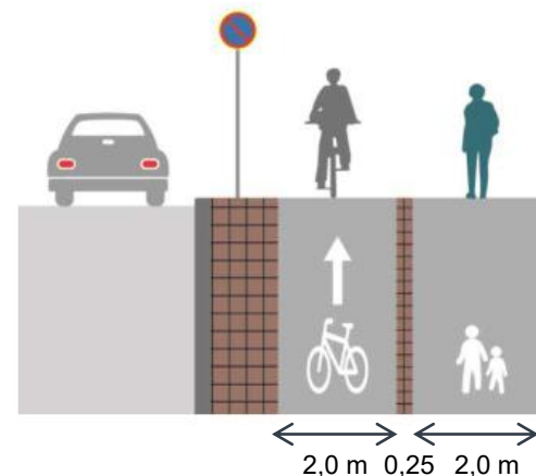
Yksisuuntainen pyörätie ja jalkakäytävä samassa tasossa
