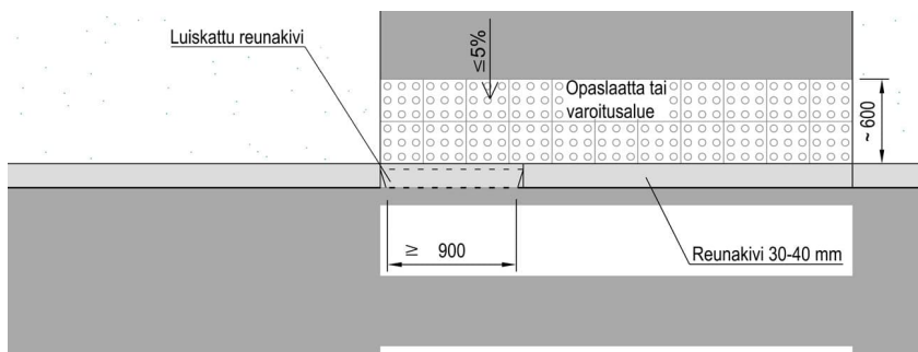
Reunatuenn asennus suojatien kohdalla. (Lähde: SuRaKu ohjekortti 1/7.)
