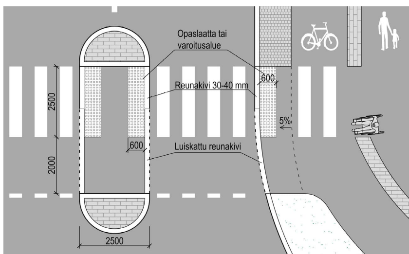
Reunatuenn asennus jalankulku- ja pyörätien kohdalla. (Lähde: SuRaKu ohjekortti 1/7.)
